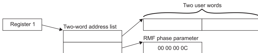
Figure 14. ERBMFTUR Input Parameter Structure
