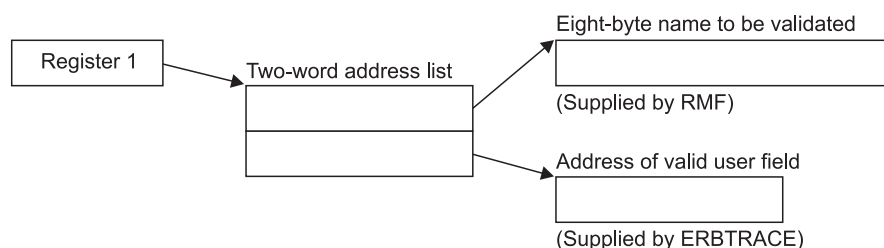
Figure 16. ERBTRACE Input Parameter Structure
