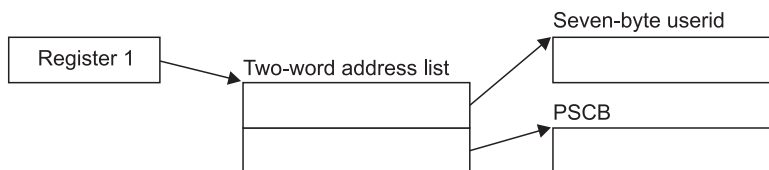
Figure 23. ERBT SOCK Input Parameter Structure
