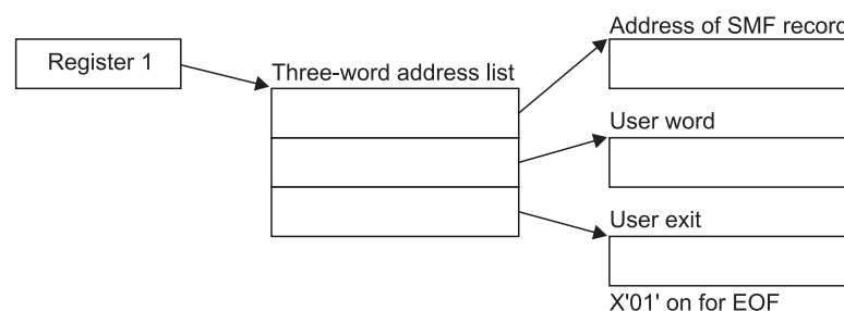
Figure 17. ERBMFPUS Input Parameter Structure
