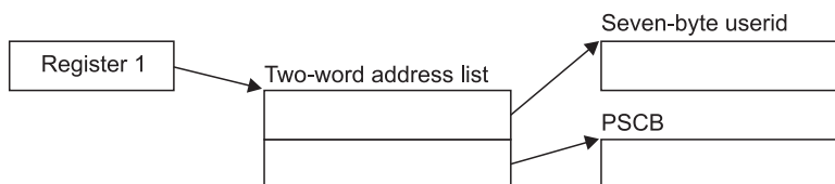
Figure 47. ERB3SOCK Input Parameter Structure
